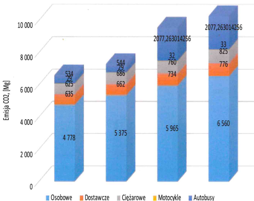
Rysunek 25 Emisja CO 2 z transportu Źródło: Opracowanie własne
