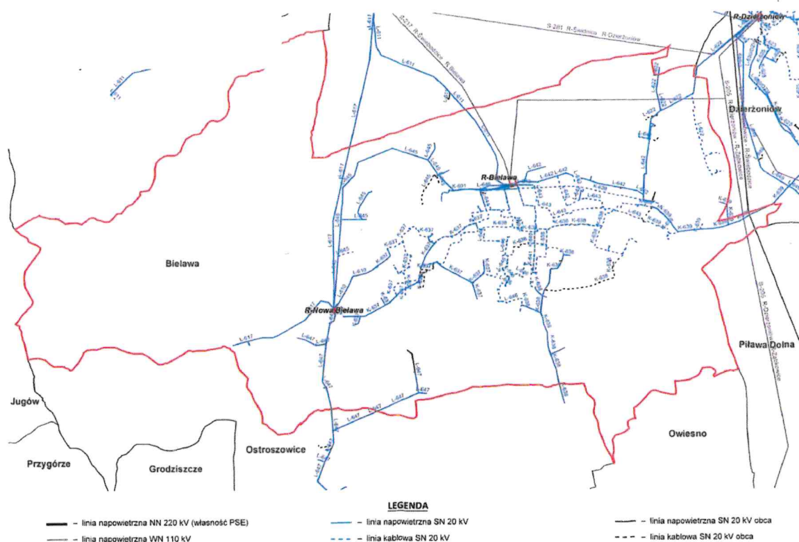
Rysunek 14 Schemat przebiegu linii WN i SN na terenie gminy Bielawa Źródło: dane pozyskane od Tauron Dystrybucja S.A.
