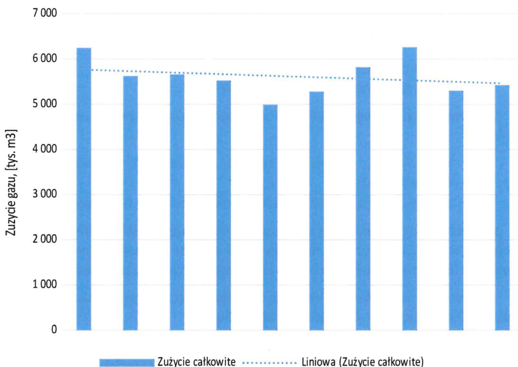
Rysunek 13 Zużycie gazu ziemnego gazu ziemnego na terenie gminy Bielawa [tys. m 3 ]
