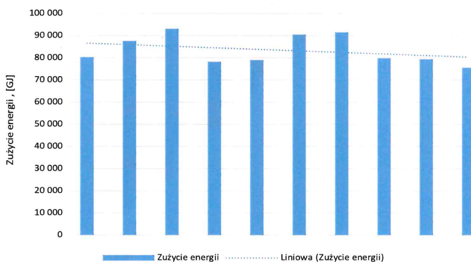
Rysunek 10 Zużycie energii ciepłej przez budynki SM Bielawa w latach 2011-2020
