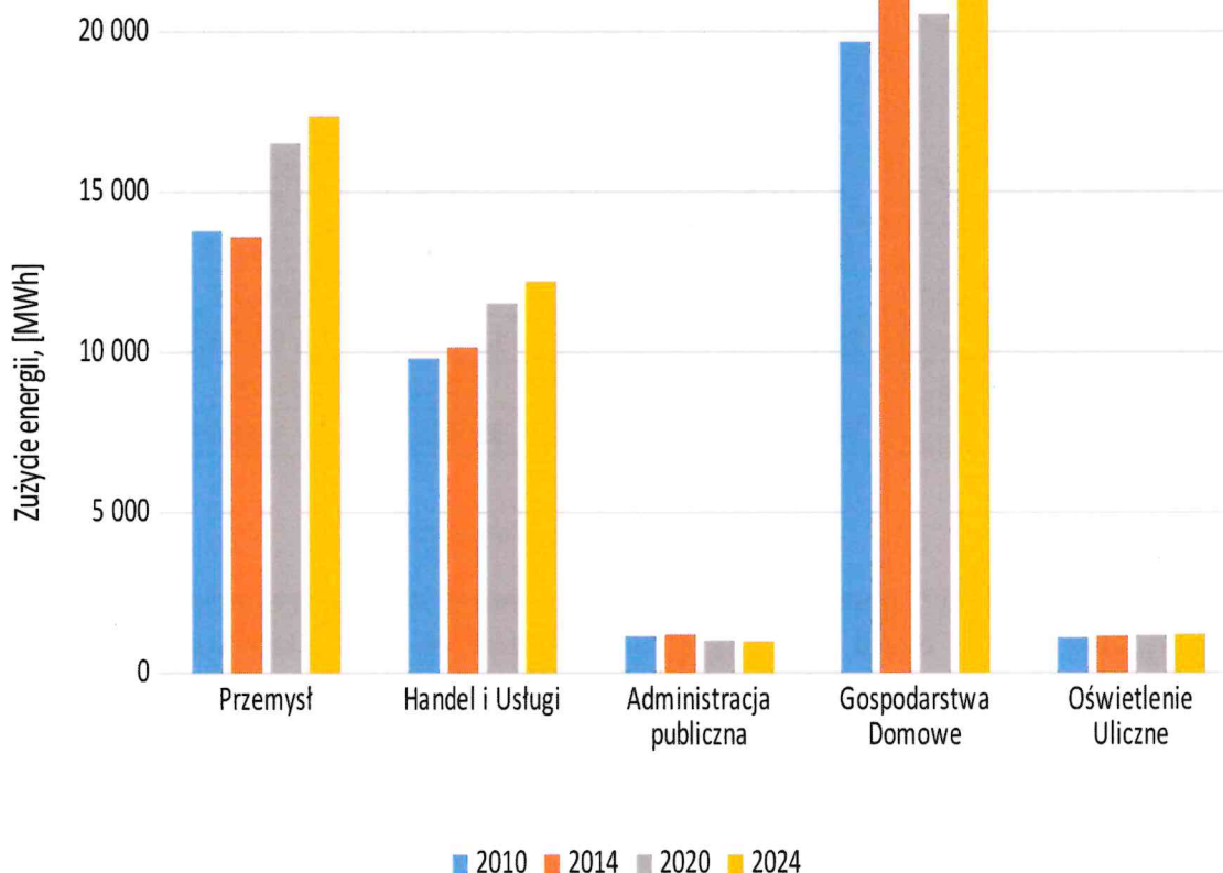
Rysunek 19 Zużycie energii przez poszczególne sektory w latach 2010 i 2014, 2020 wraz z prognozą na rok 2024 Źródło: Opracowanie własne
